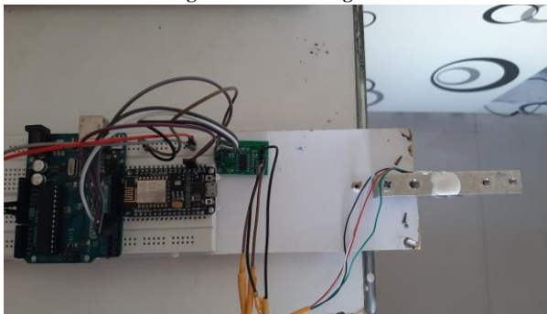
Figure 5. Actual Circuit
